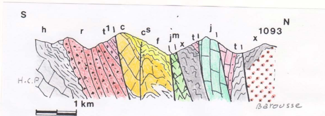
Figure 4B : Coupe géologique (d'après C. Lucas) en rive gauche de la Neste. Les terrains exploités sont représentés en jaune et notés C. Ils affleurent au Nord des terrains (couleurs rouge et rose, notés r1 et r2) du Permo-trias (appartenant à la couverture de la Haute chaîne Primaire) avec lesquels ils sont en contact par faille et au Sud des terrains notés Jm représentés par une couleur verte ; là aussi le contact est une faille.
