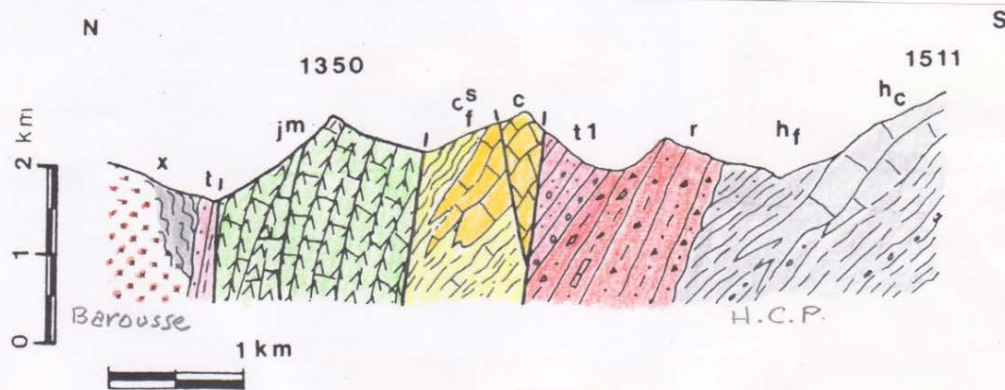
Figure 4C : Coupe géologique (d'après C. Lucas) en rive droite de la Neste. La disposition est identique à la coupe précédente. Le contact est par faille au Sud avec le Permo-trias (faille Nord pyrénéenne que nous observerons sur le chemin de Castet) et avec le Jurassique métamorphique.
