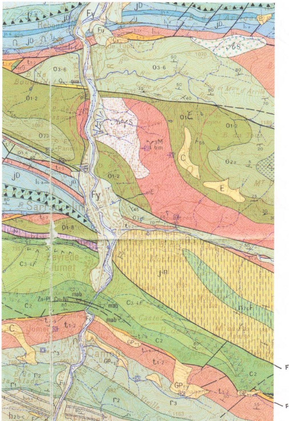
Figure 4A : Extrait de la carte géologique d'Arreau au 1/50000, BRGM. Les carrières se situent au Sud de Sarrancolin dans les secteurs de Beyrède-Jumet (rive gauche de la Neste) et d'Ilhet (rive droite de la Neste), dans une étroite bande de terrains représentés en vert et notés C2, limitée par deux failles grossièrement Ouest-Est.
