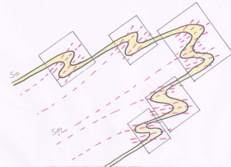
Figure 3A : Schéma d'un pli complexe montrant la localisation de la structure griotte (rectangles). S0 est la stratification et Sm la schistosité.
