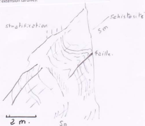
Figure 3B : Pli décramétrique dans la carrière d'Espiadet d'extension tardives.
